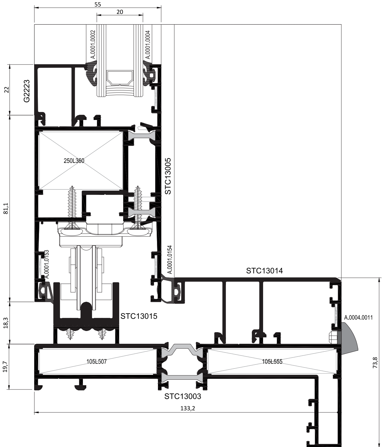
ÇEK-SÜR DETAYI PULL & SLIDE DETAIL
