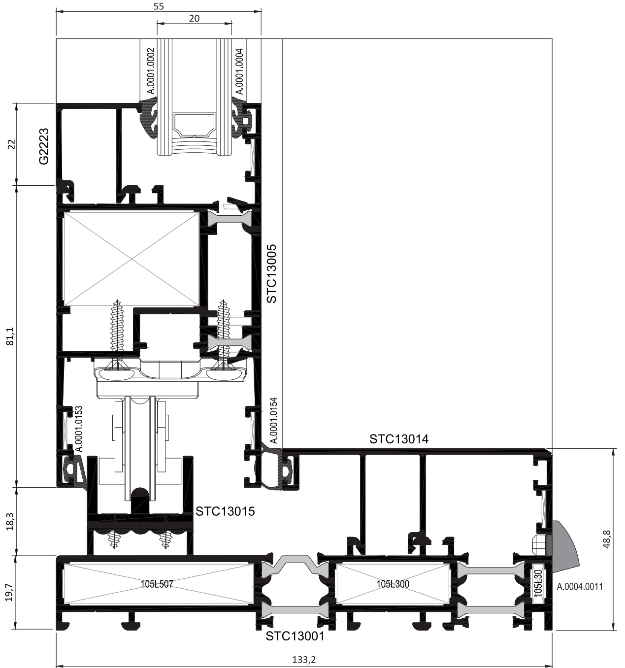
ÇEK-SÜR DETAYI PULL & SLIDE DETAIL
