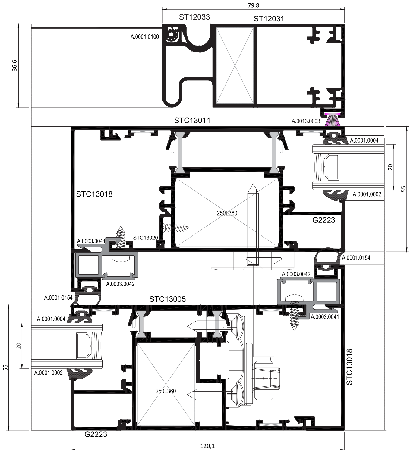
ÇEK-SÜR DETAYI PULL & SLIDE DETAIL
