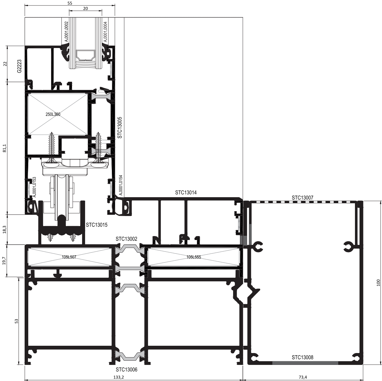
ÇEK-SÜR DETAYI PULL & SLIDE DETAIL
