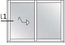
ÇEK-SÜR DETAYI PULL & SLIDE DETAIL
