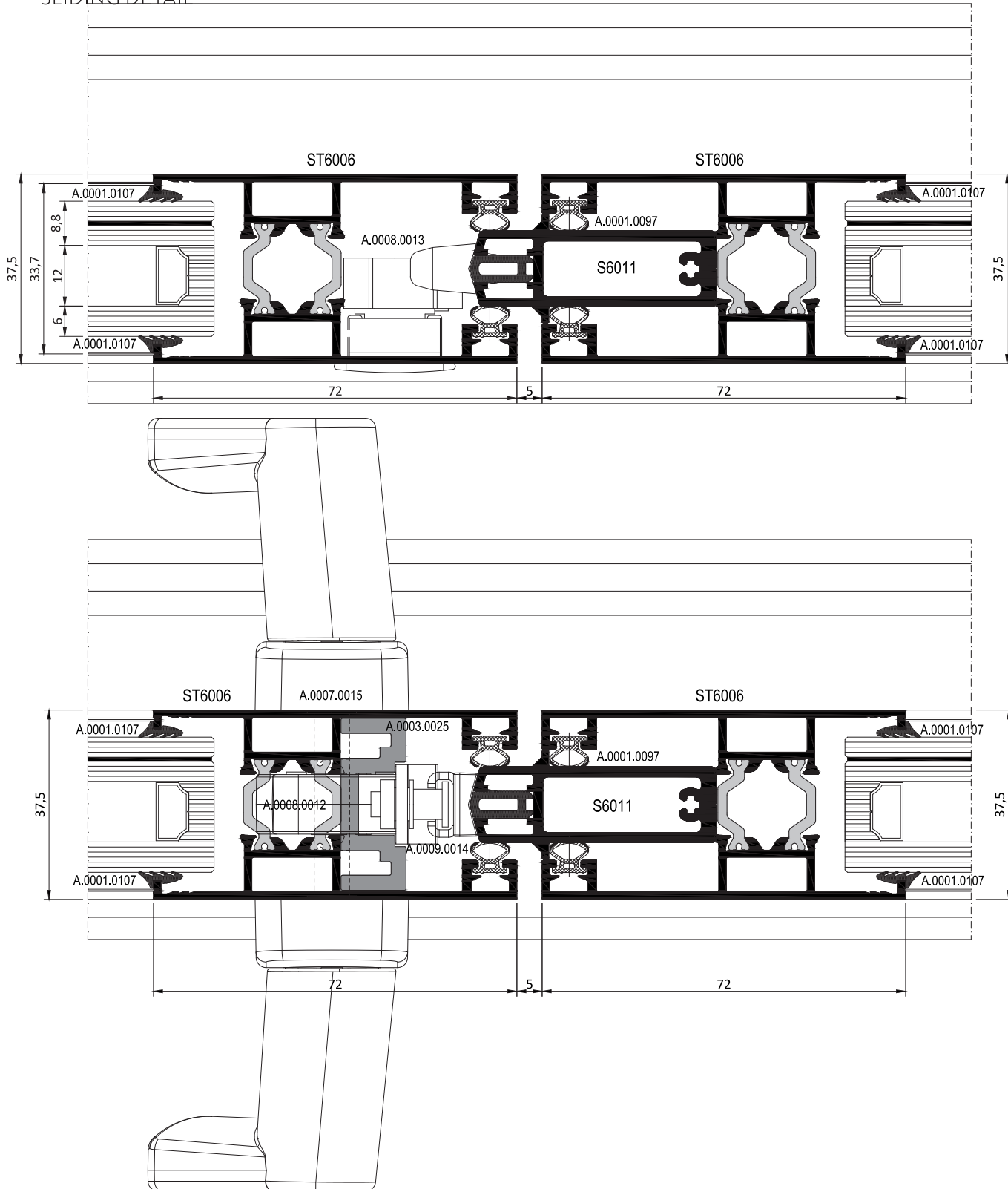
SÜRME DETAYI SLIDING DETAIL
