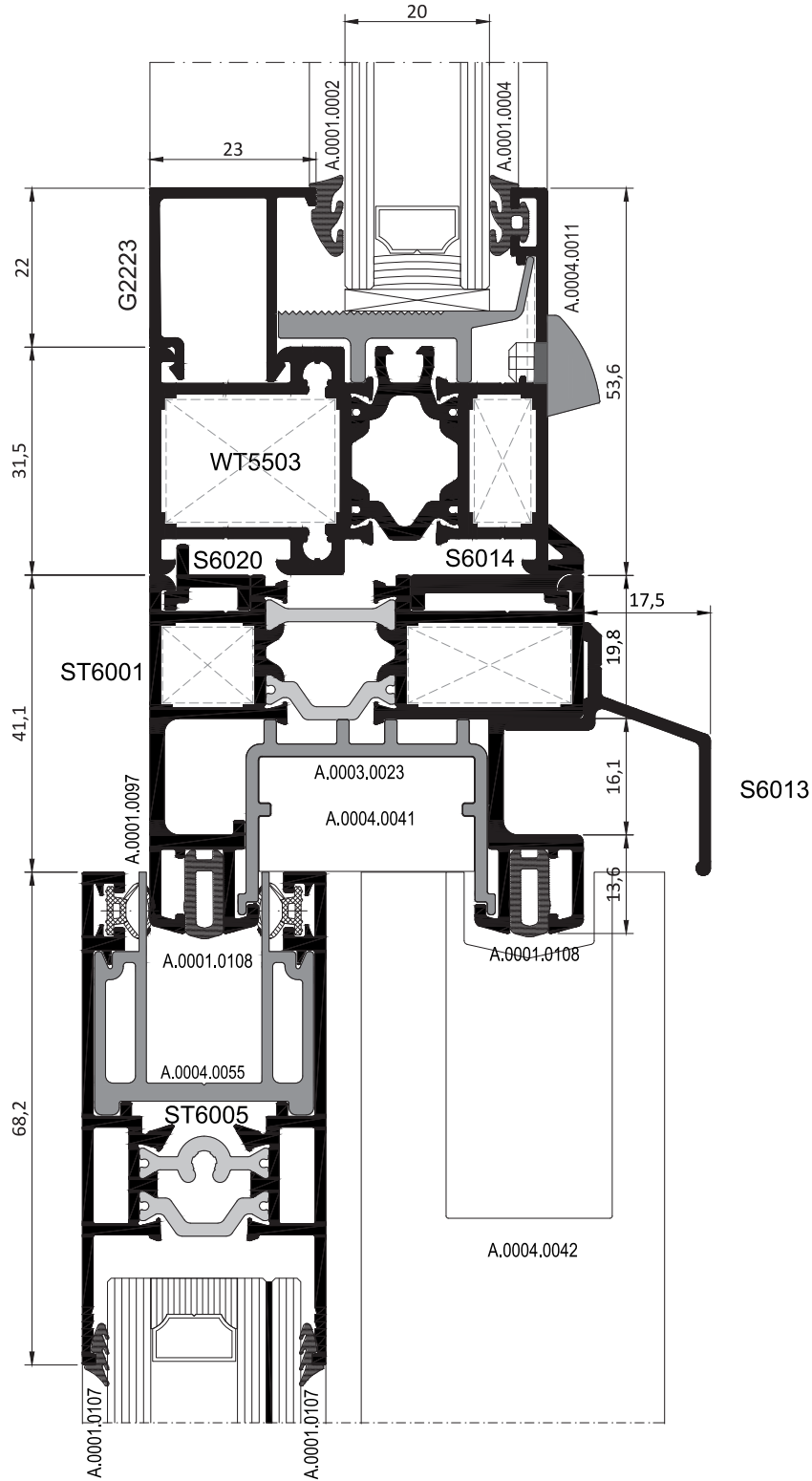
SÜRME DETAYI SLIDING DETAIL
