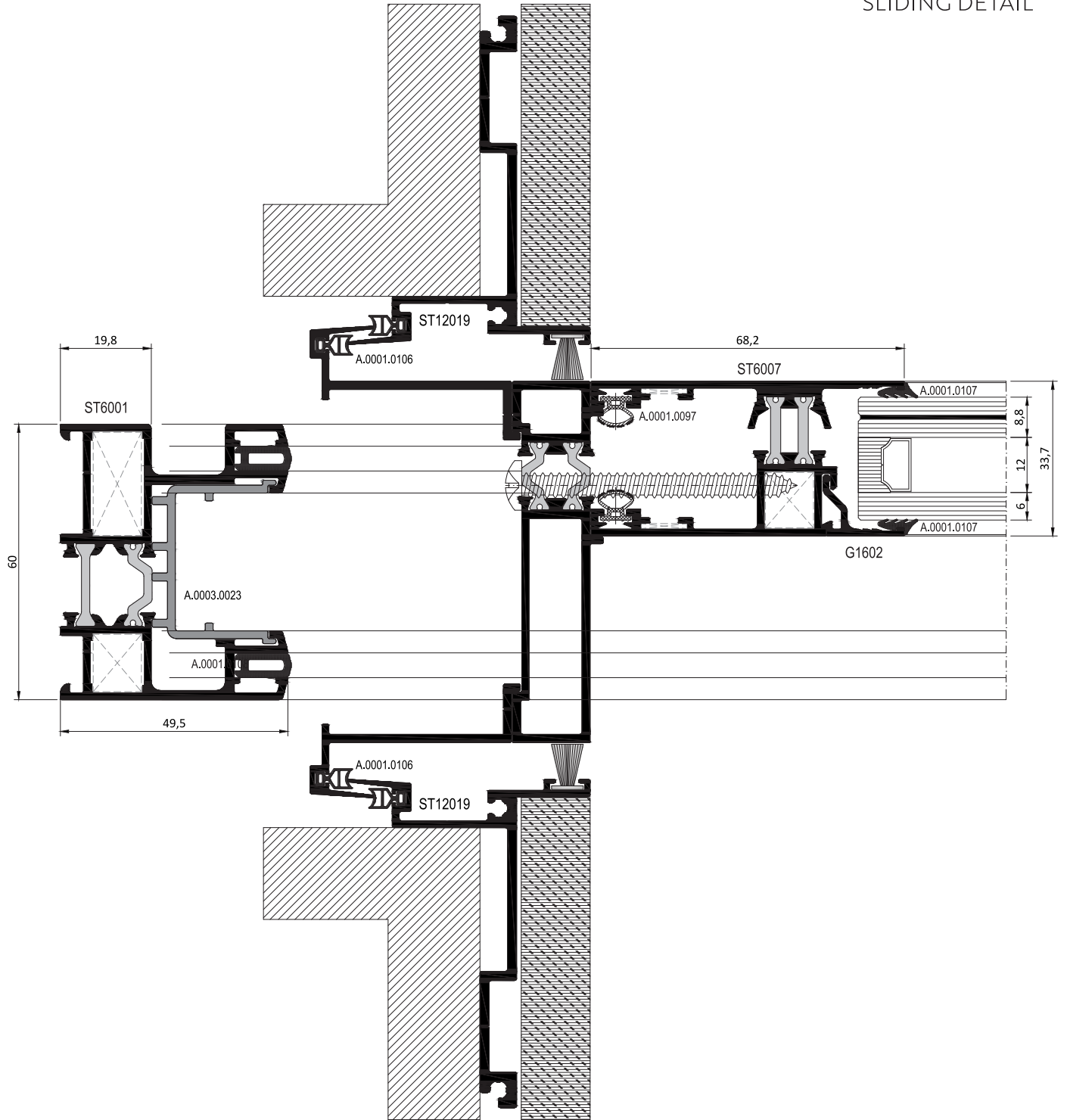
SÜRME DETAYI SLIDING DETAIL
