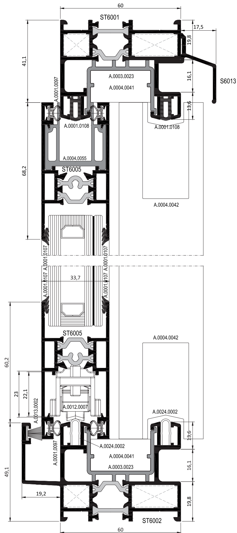
SÜRME DETAYI SLIDING DETAIL
