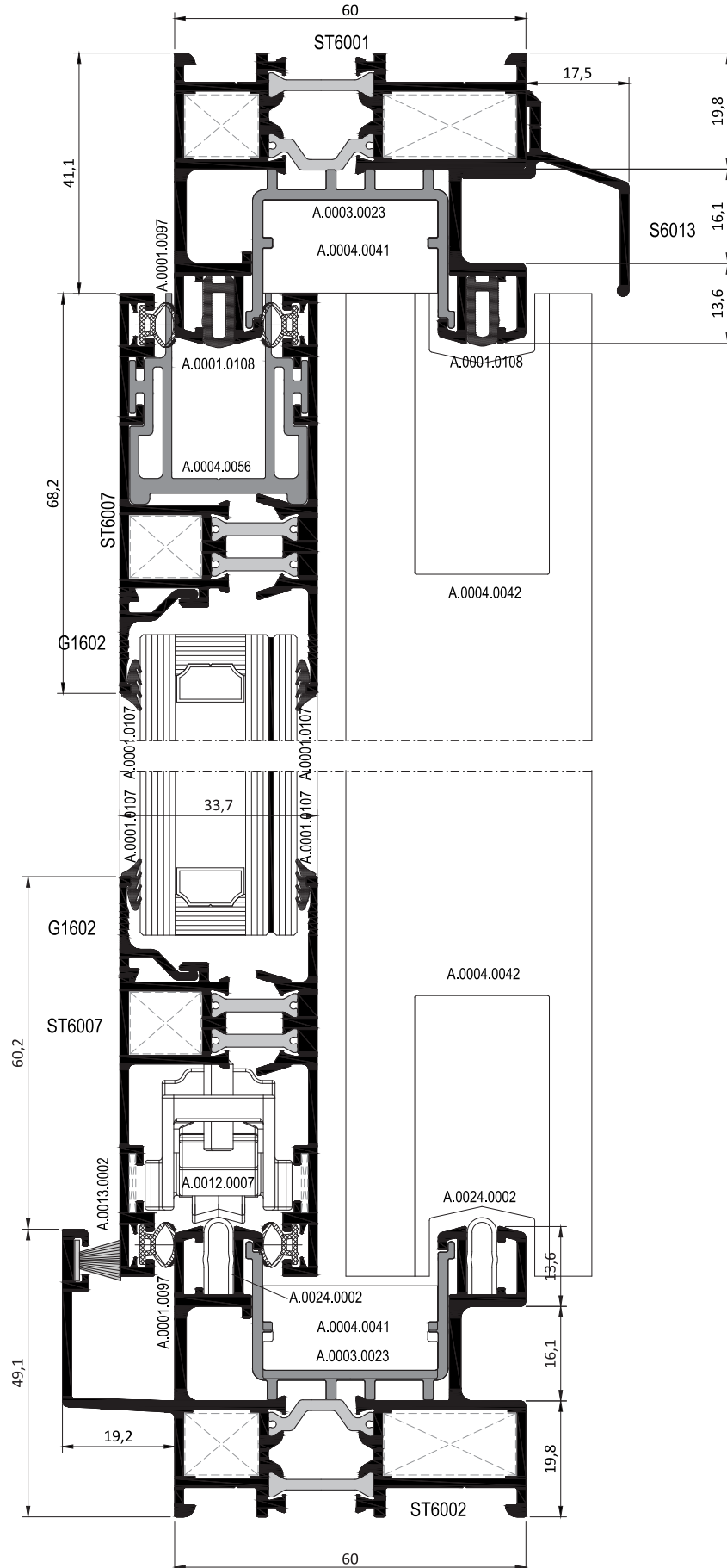
SÜRME DETAYI SLIDING DETAIL
