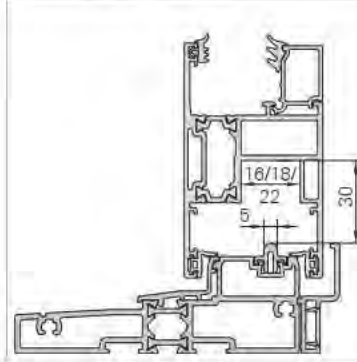
Slim varyantları için kanal / Groove for Slim version
