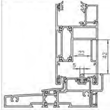
Strok gösterimi / Trave illustration
