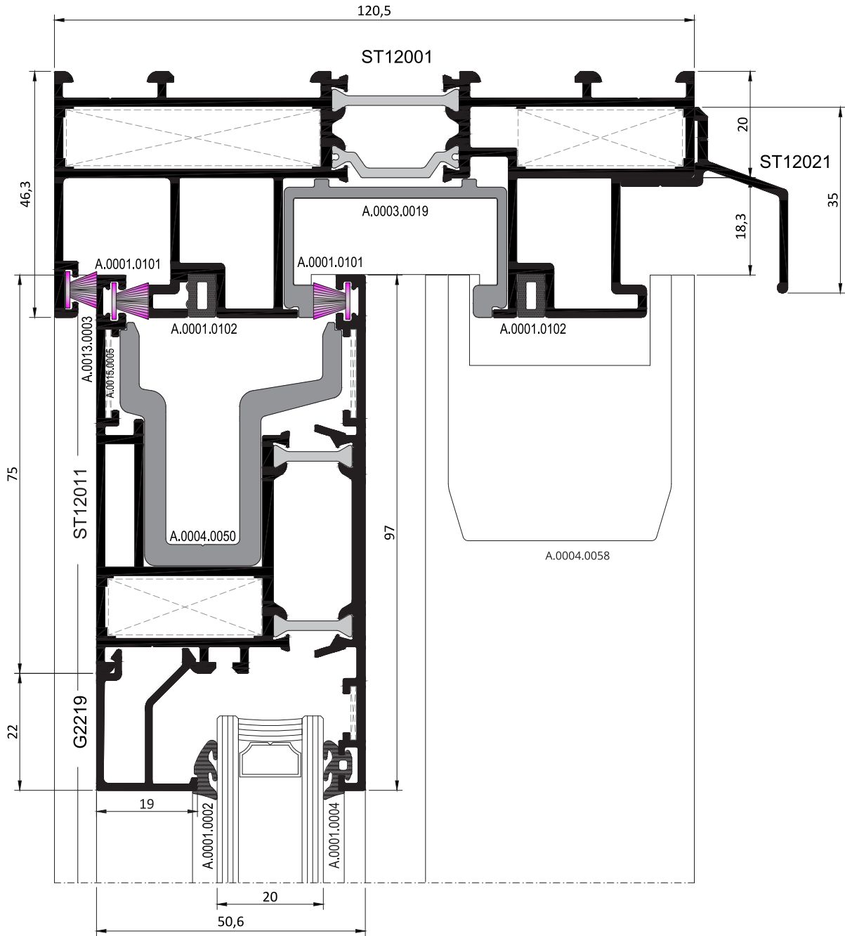
SÜRME DETAYI SLIDING DETAIL
