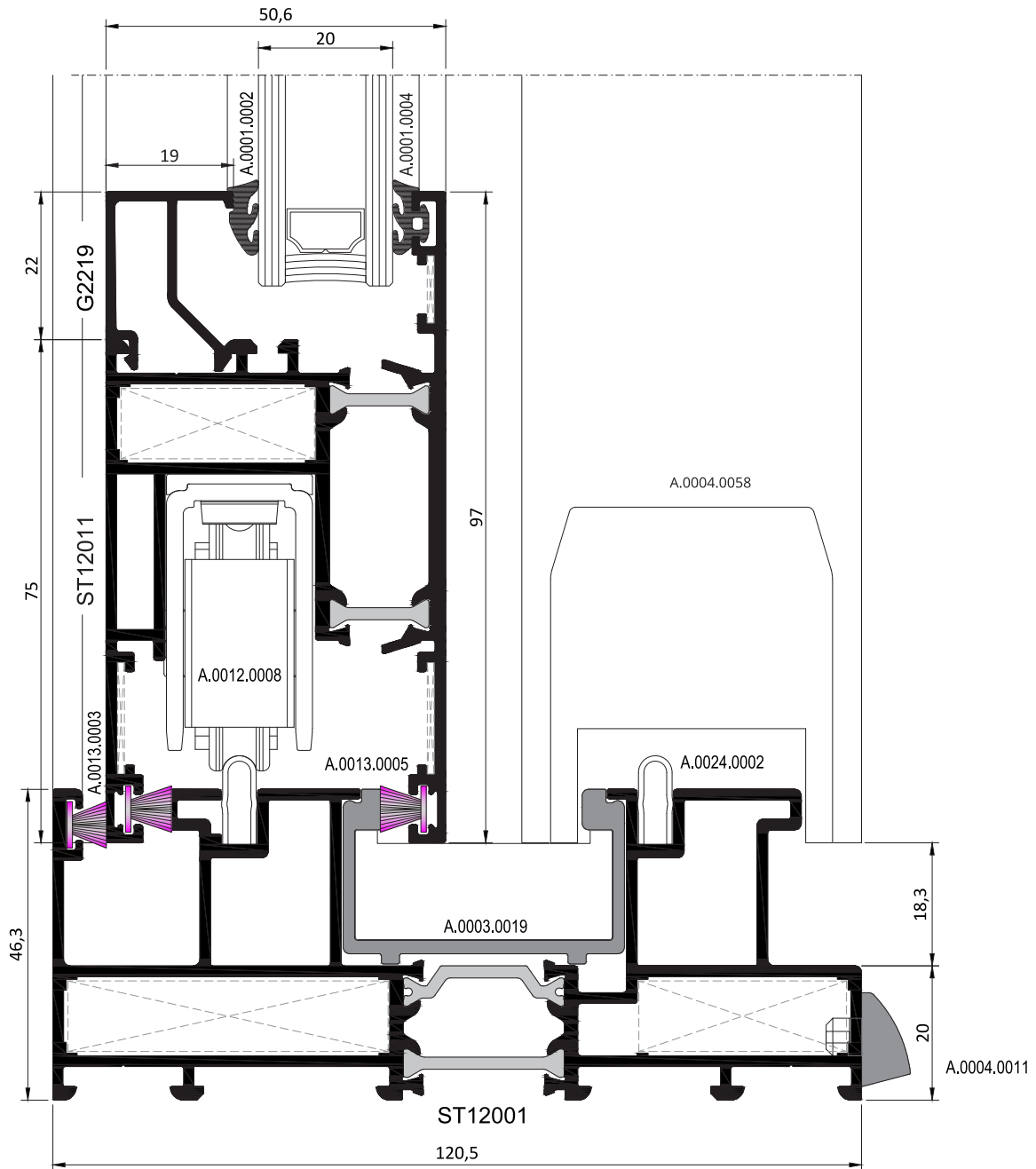
SÜRME DETAYI SLIDING DETAIL
