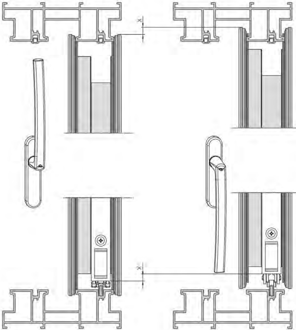
Strok gösterimi / Trave illustration
