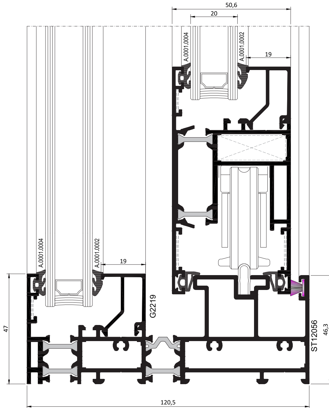
SÜRME DETAYI SLIDING DETAIL
