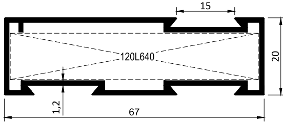
Kod / Code : S6701 Profil No / Profile No : P11400 Ağırlık / Weight : 0.657 kg/m
