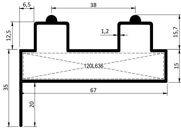
Kod / Code : S6704 Profil No / Profile No : P11403 Ağırlık / Weight : 0.807 kg/m
