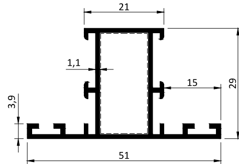
Kod / Code : S6704 Profil No / Profile No : P11403 Ağırlık / Weight : 0.807 kg/m
