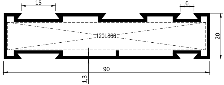
Kod / Code : S6702 Profil No / Profile No : P11401 Ağırlık / Weight : 0.899 kg/m
