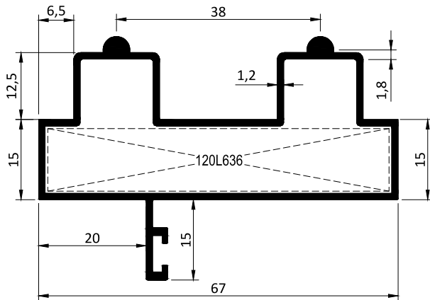
Kod / Code : S6705 Profil No / Profile No : P11404 Ağırlık / Weight : 0.821 kg/m
