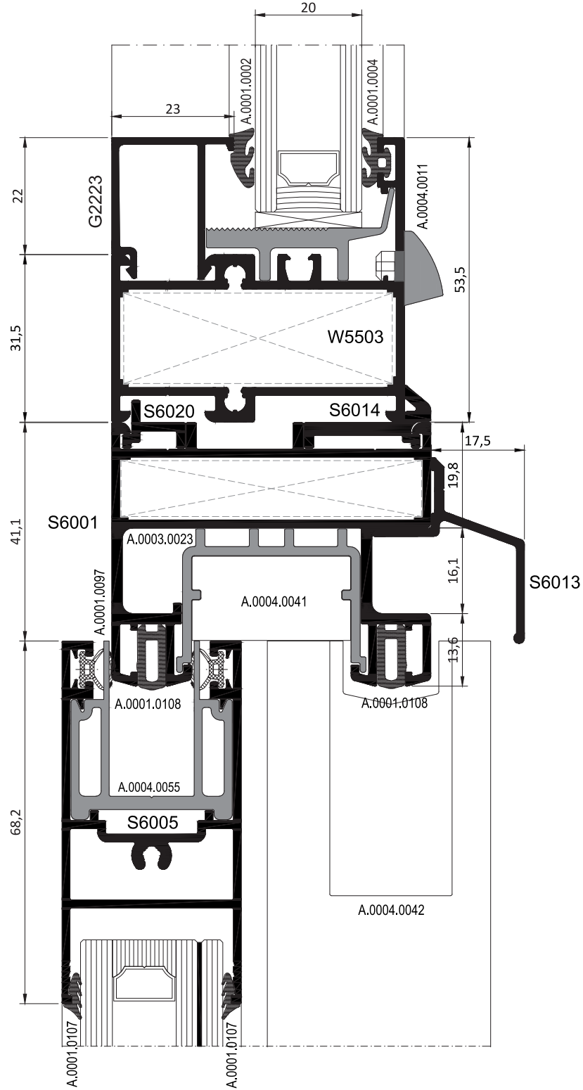
SÜRME DETAYI SLIDING DETAIL
