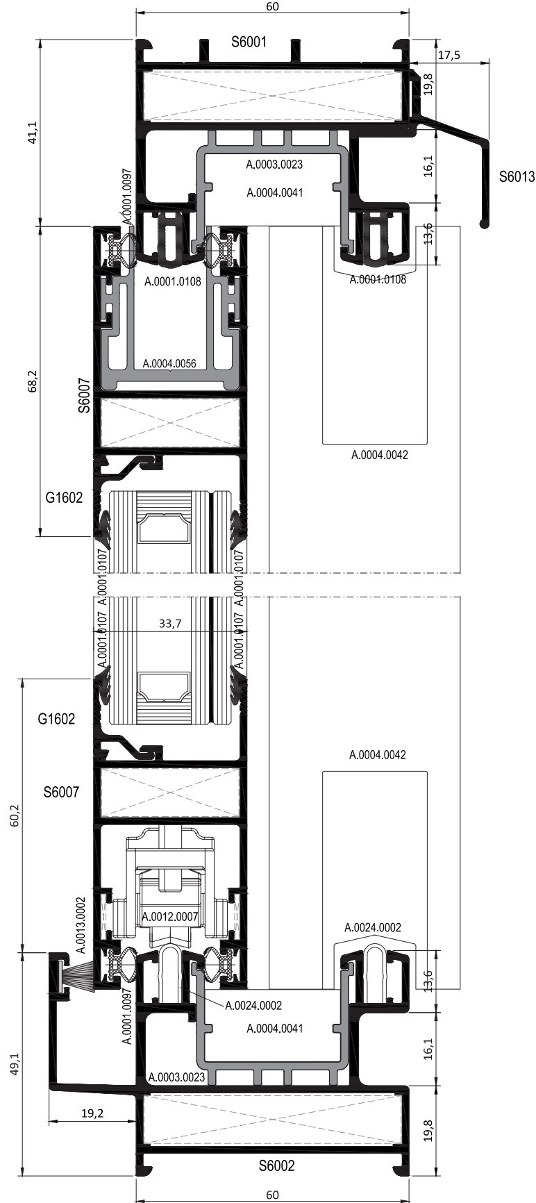
SÜRME DETAYI SLIDING DETAIL
