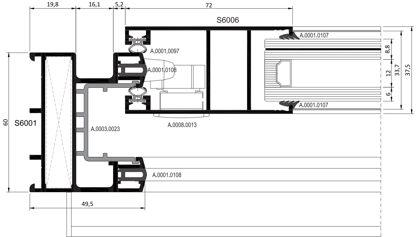
SÜRME DETAYI SLIDING DETAIL
