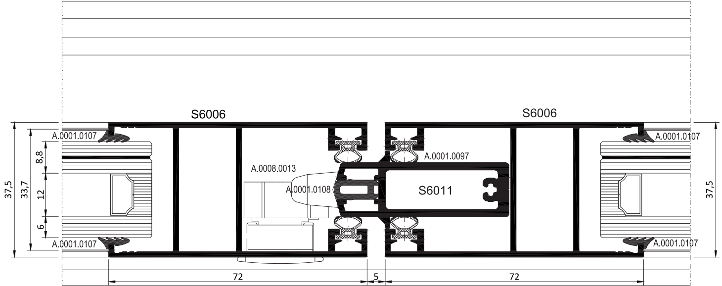
SÜRME DETAYI SLIDING DETAIL
