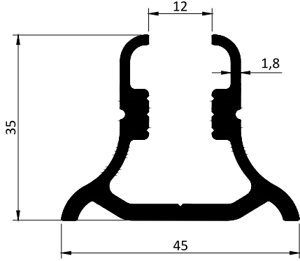
Kod / Code : P10042 Ağırlık / Weight : 0.906 kg/m
