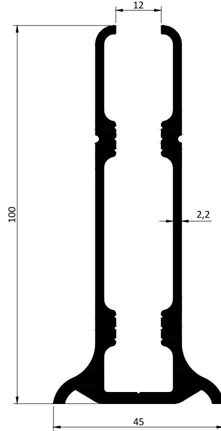
Kod / Code : P10045 Ağırlık / Weight : 2.031 kg/m
