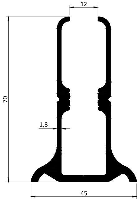
Kod / Code : P10044 Ağırlık / Weight : 1.384 kg/m
