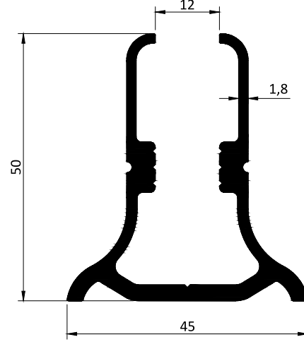
Kod / Code : P10043 Ağırlık / Weight : 1.057 kg/m
