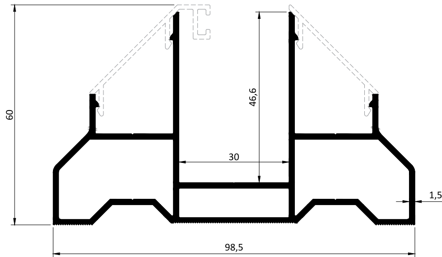
Kod / Code : P10046 Profil No / Profile No : P10046 Ağırlık / Weight : 1.493 kg/m
