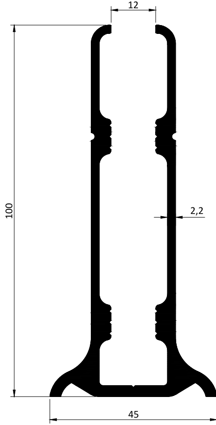
Kod / Code : P10045 Profil No / Profile No : P10045 Ağırlık / Weight : 2.031 kg/m
