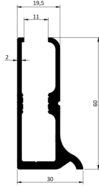
Kod / Code : P10081 Profil No / Profile No : P10081 Ağırlık / Weight : 1.069 kg/m
