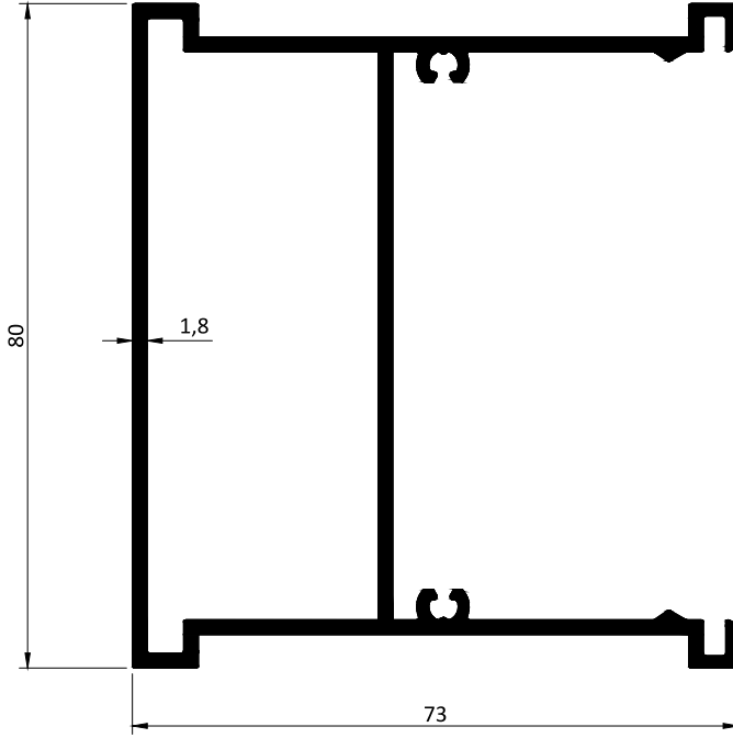
Kod / Code : O7504 Profil No / Profile No : P11524 Ağırlık / Weight : 1.602 kg/m
