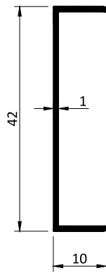
Kod / Code : O2514 Profil No / Profile No : P11513 Ağırlık / Weight : 0.163 kg/m
