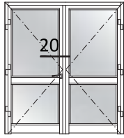
ÇİFT KANAT DIŞA AÇILIM BİNİLİ KAPI DETAYI OUTWARD OPENING DOUBLE VENT DOOR DETAIL
