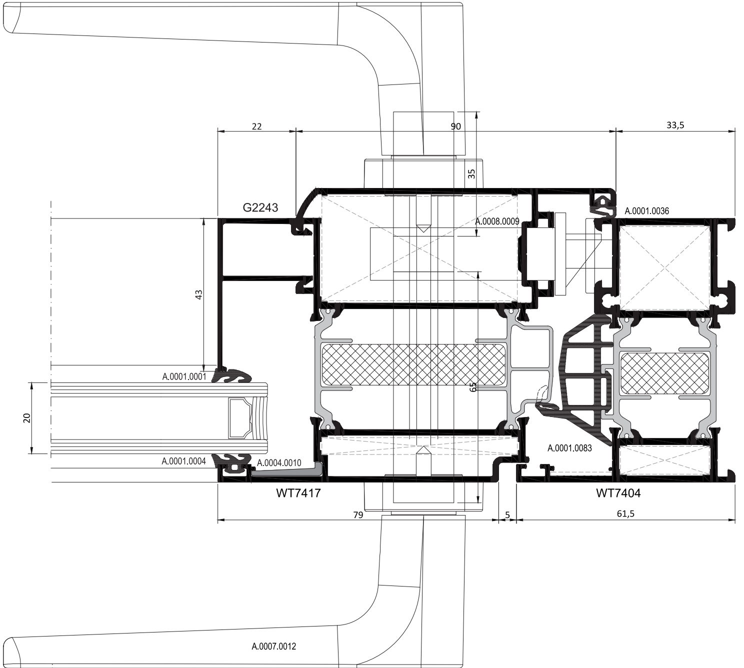
İÇE AÇILIM BİNLİ KAPI DETAYI INWARD OPENING DOOR DETAIL
