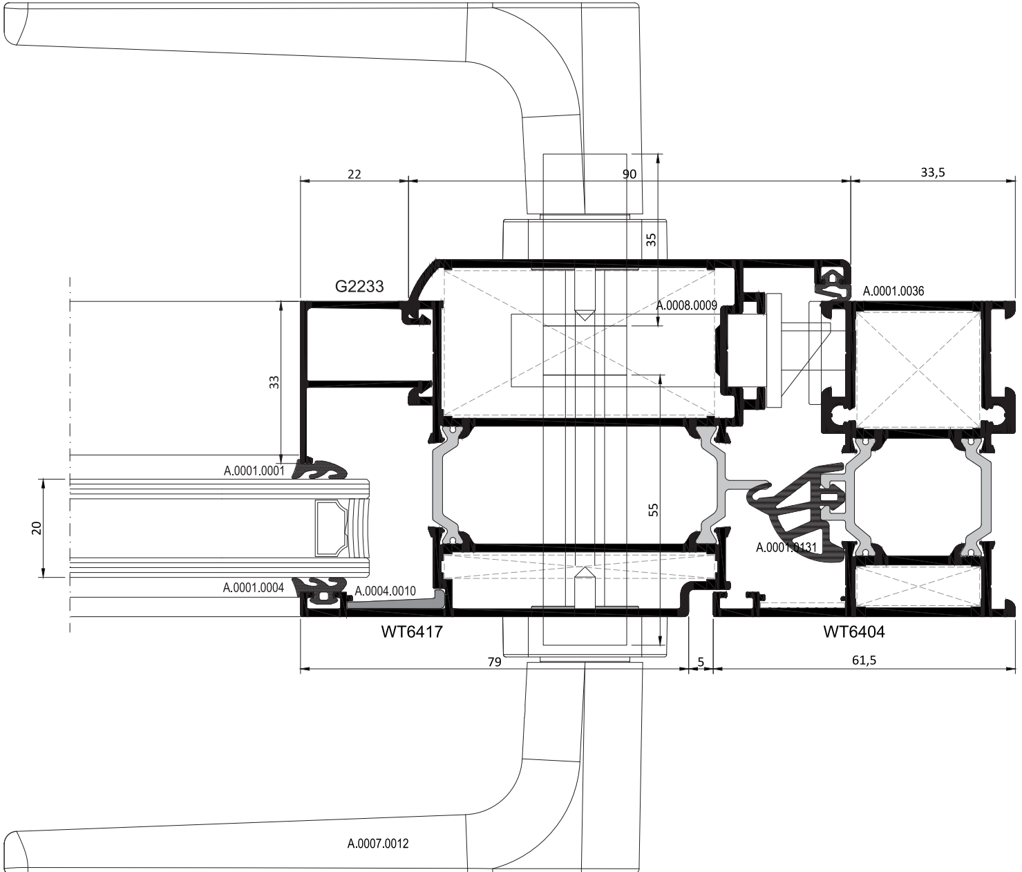
İÇE AÇILIM BİNLİ KAPI DETAYI INWARD OPENING DOOR DETAIL
