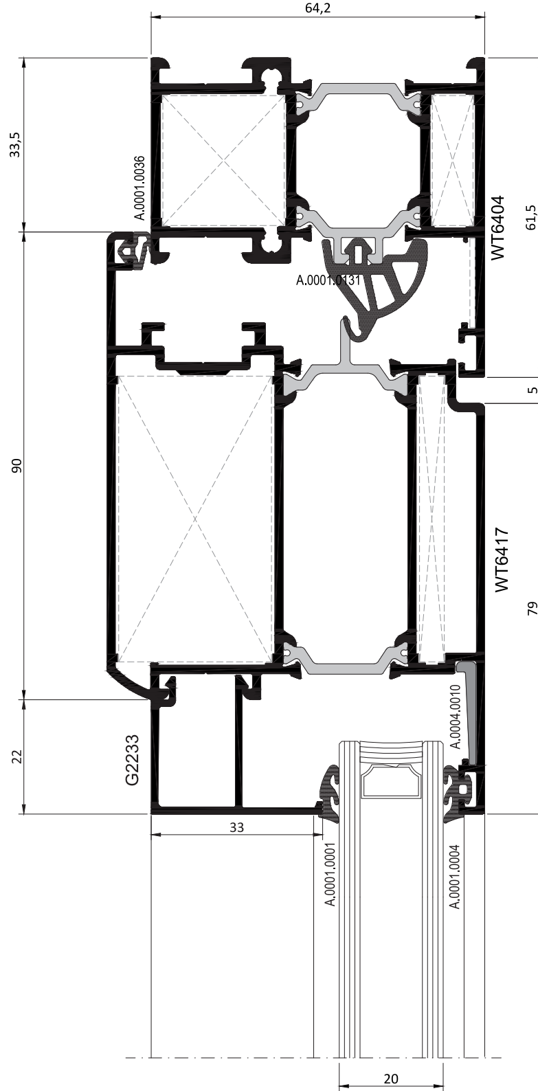
İÇE AÇILIM BİNLİ KAPI DETAYI INWARD OPENING DOOR DETAIL
