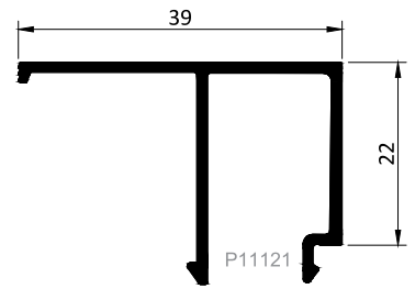
Kod / Code : G2239 Profil No / Profile No : P11121 Ağırlık / Weight : 0.334 kg/m
