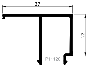
Kod / Code : G2237 Profil No / Profile No : P11120 Ağırlık / Weight : 0.327 kg/m
