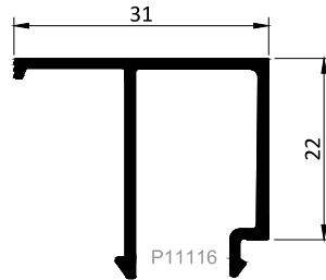
Kod / Code : G2231 Profil No / Profile No : P11116 Ağırlık / Weight : 0.308 kg/m
