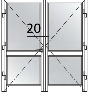
ÇİFT KANAT DIŞA AÇILIM BİNLİ KAPI DETAYI OUTWARD OPENING DOUBLE VENT DOOR DETAIL
