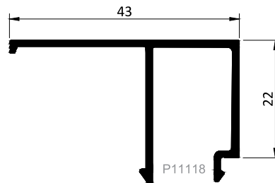
Kod / Code : G2243 Profil No / Profile No : P11118 Ağırlık / Weight : 0.347 kg/m
