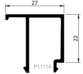
Kod / Code : G2227 Profil No / Profile No : P11114 Ağırlık / Weight : 0.294 kg/m
