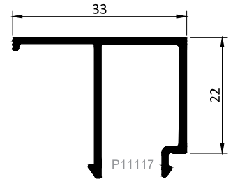
Kod / Code : G2233 Profil No / Profile No : P11117 Ağırlık / Weight : 0.314 kg/m
