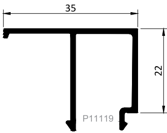
Kod / Code : G2235 Profil No / Profile No : P11119 Ağırlık / Weight : 0.321 kg/m
