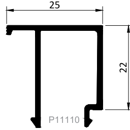
Kod / Code : G2225 Profil No / Profile No : P11110 Ağırlık / Weight : 0.288 kg/m
