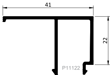
Kod / Code : G2241 Profil No / Profile No : P11122 Ağırlık / Weight : 0.340 kg/m
