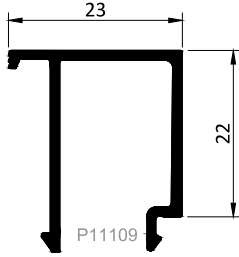
Kod / Code : G2223 Profil No / Profile No : P11109 Ağırlık / Weight : 0.282 kg/m
