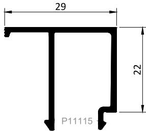
Kod / Code : G2229 Profil No / Profile No : P11115 Ağırlık / Weight : 0.301 kg/m
