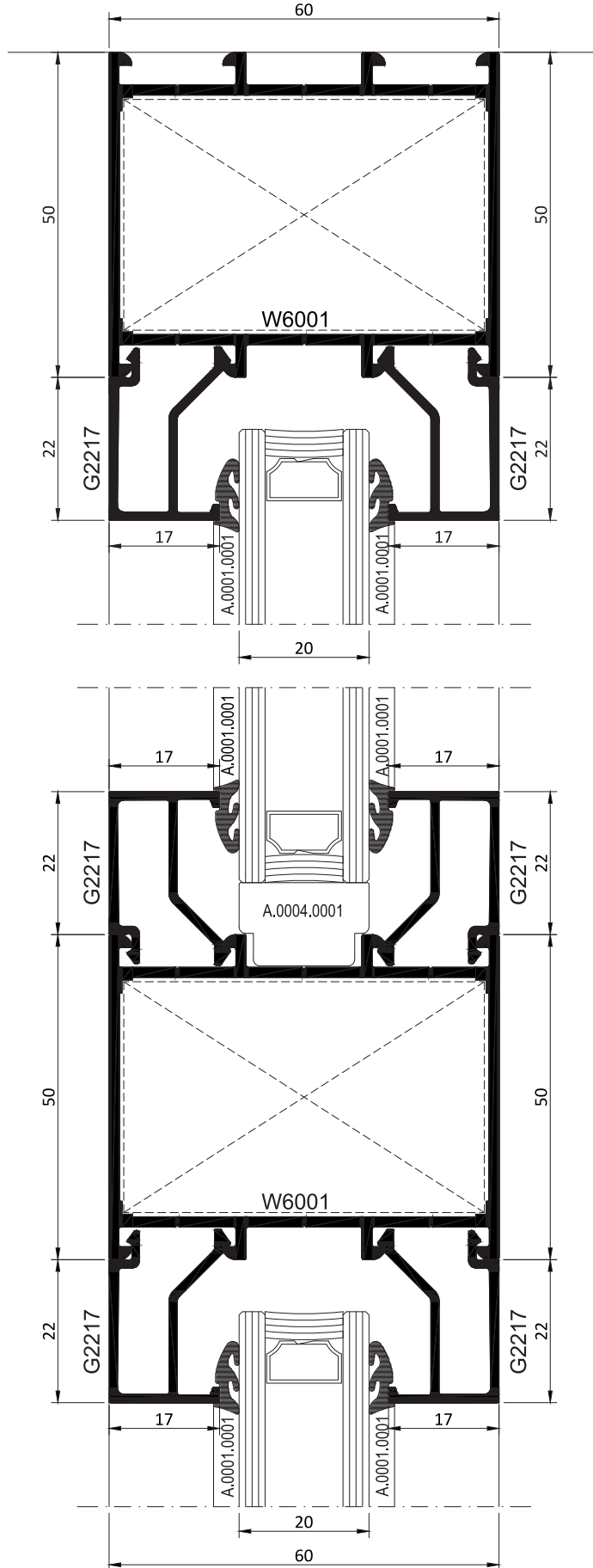
ÇİFT KANAT KAPI DOUBLE VENT DOOR
