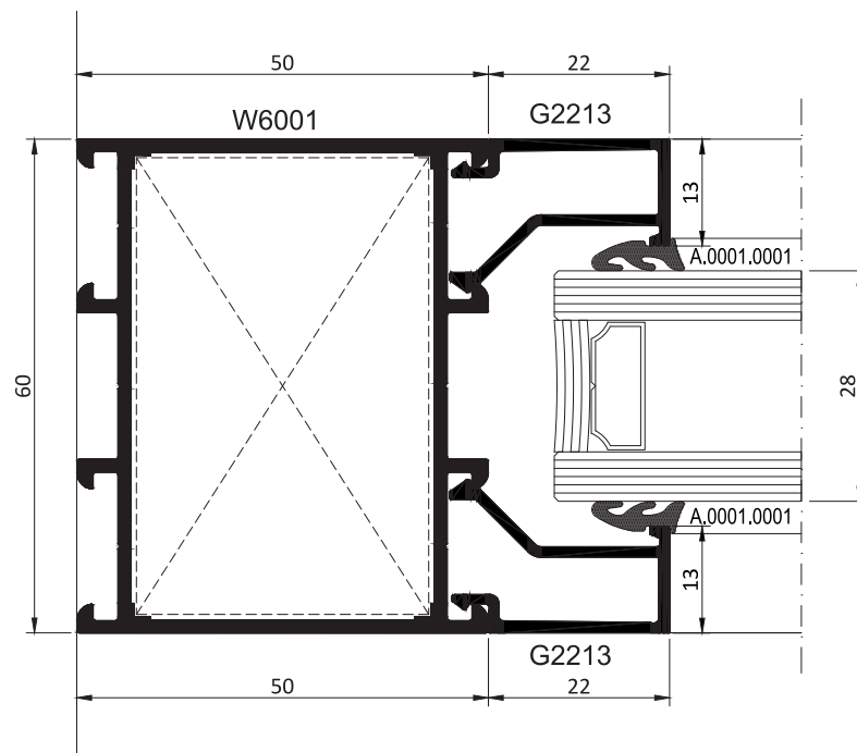
ÇİFT KANAT KAPI DOUBLE VENT DOOR
