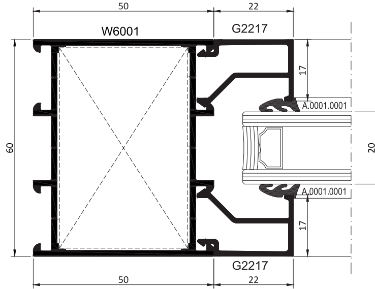
ÇİFT KANAT KAPI DOUBLE VENT DOOR
