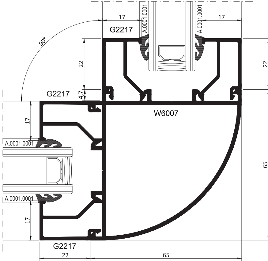
90° DÖNÜŞ 90° CORNER
