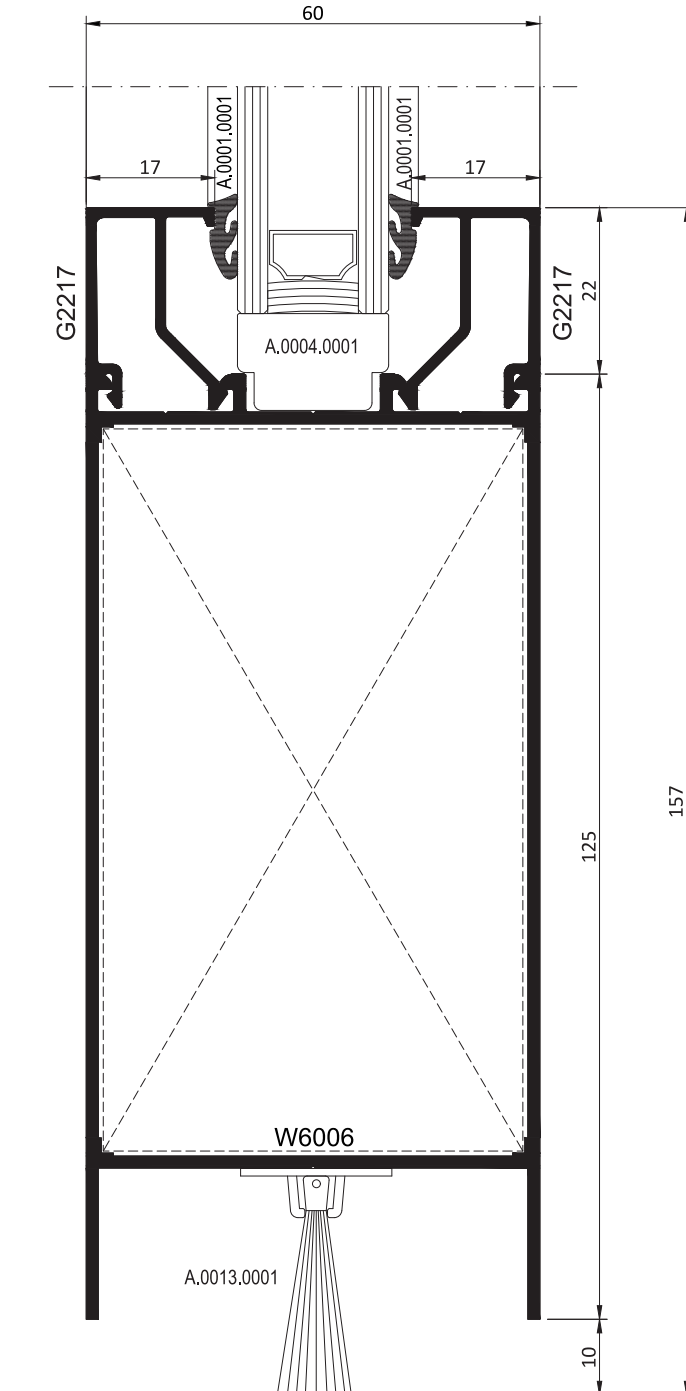
ÇARPMA KANAT KAPI SWINGING VENT DOOR
