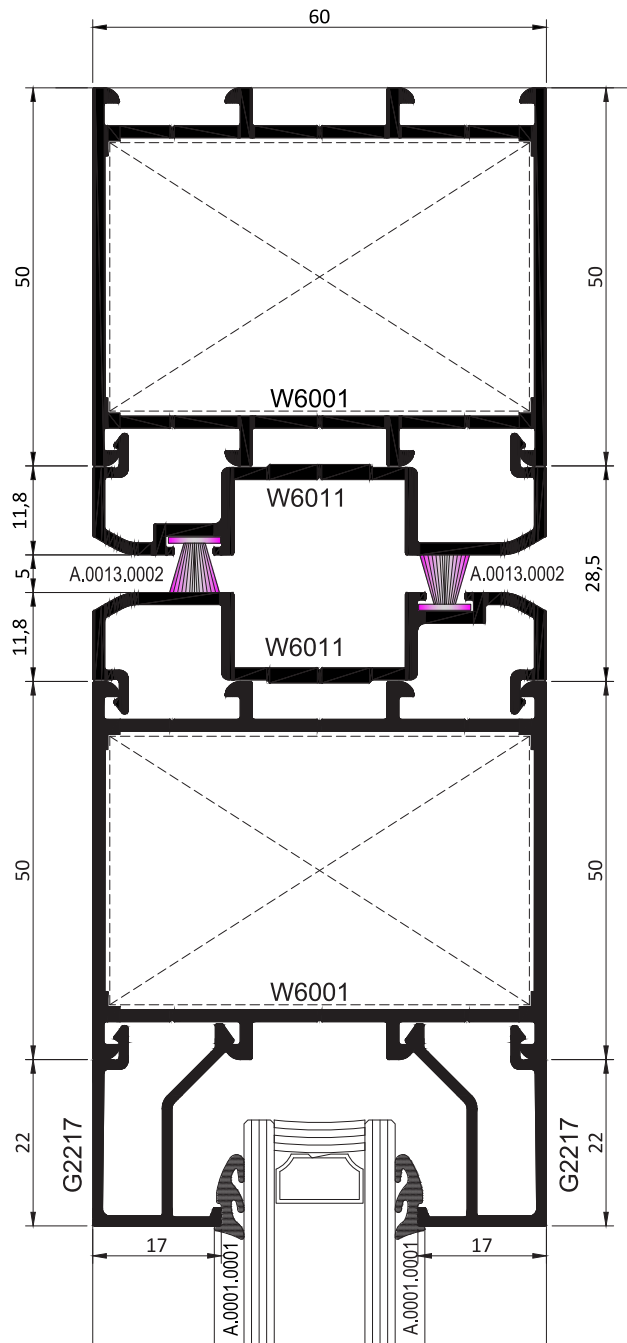
ÇARPMA KANAT KAPI SWINGING VENT DOOR
