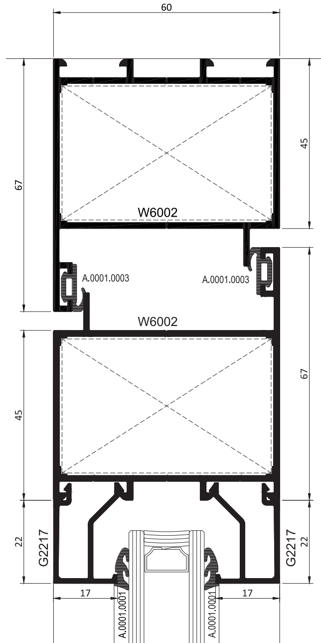
TEK KANAT KAPI SINGLE VENT DOOR
