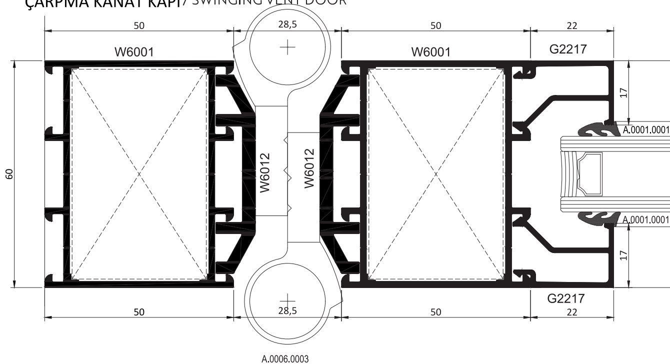
ÇARPMA KANAT KAPI / SWINGING VENT DOOR
