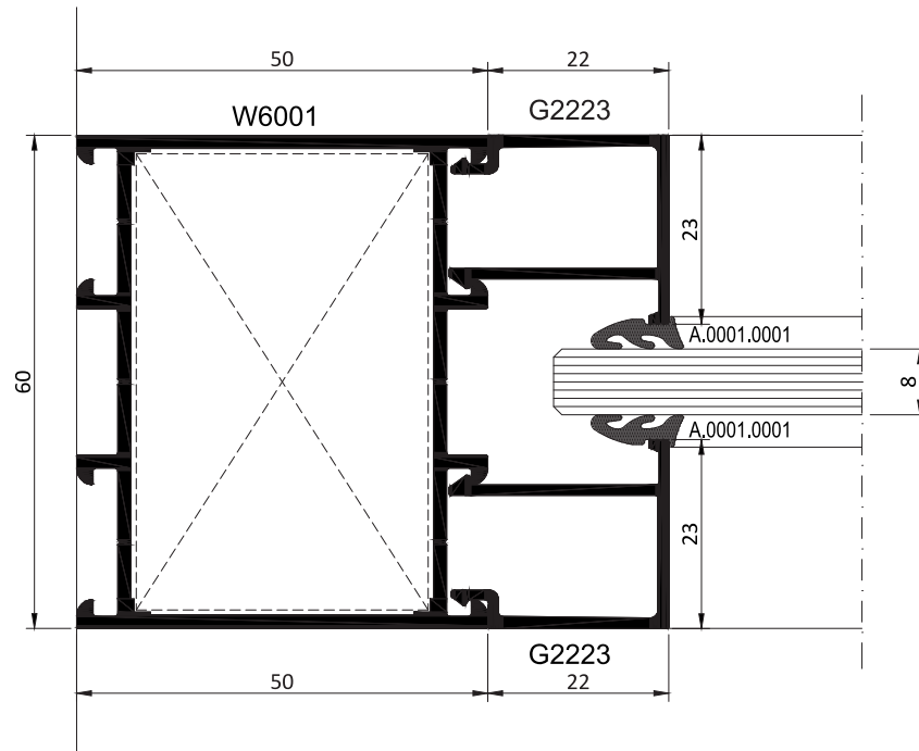
ÇİFT KANAT KAPI DOUBLE VENT DOOR
