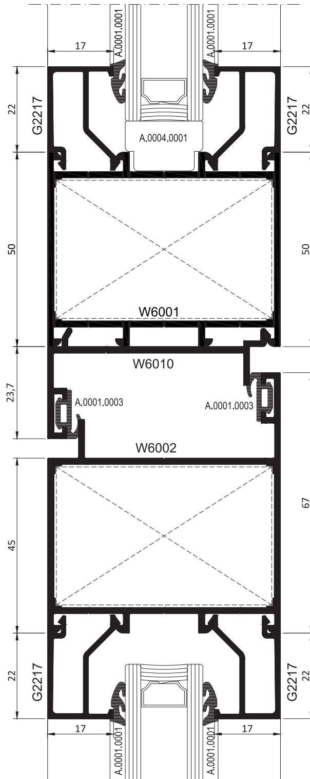
ÇİFT KANAT KAPI DOUBLE VENT DOOR
