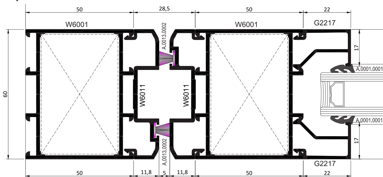
ÇARPMA KANAT KAPI / SWINGING VENT DOOR
