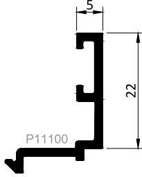
Kod / Code : G2205 Profil No / Profile No : P11100 Ağırlık / Weight : 0.220 kg/m
