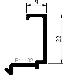
Kod / Code : G2209 Profil No / Profile No : P11102 Ağırlık / Weight : 0.206 kg/m
