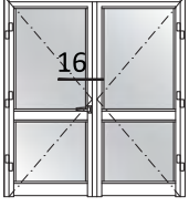
ÇİFT KANAT İÇE AÇILIM BİNLİ KAPI DETAYI INWARD OPENING DOUBLE VENT DOOR DETAIL
