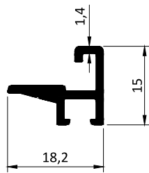
Kod / Code : WT6453 Profil No / Profile No : P13050 Ağırlık / Weight : 0.189 kg/m
