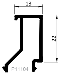
Kod / Code : G2213 Profil No / Profile No : P11104 Ağırlık / Weight : 0.257 kg/m
