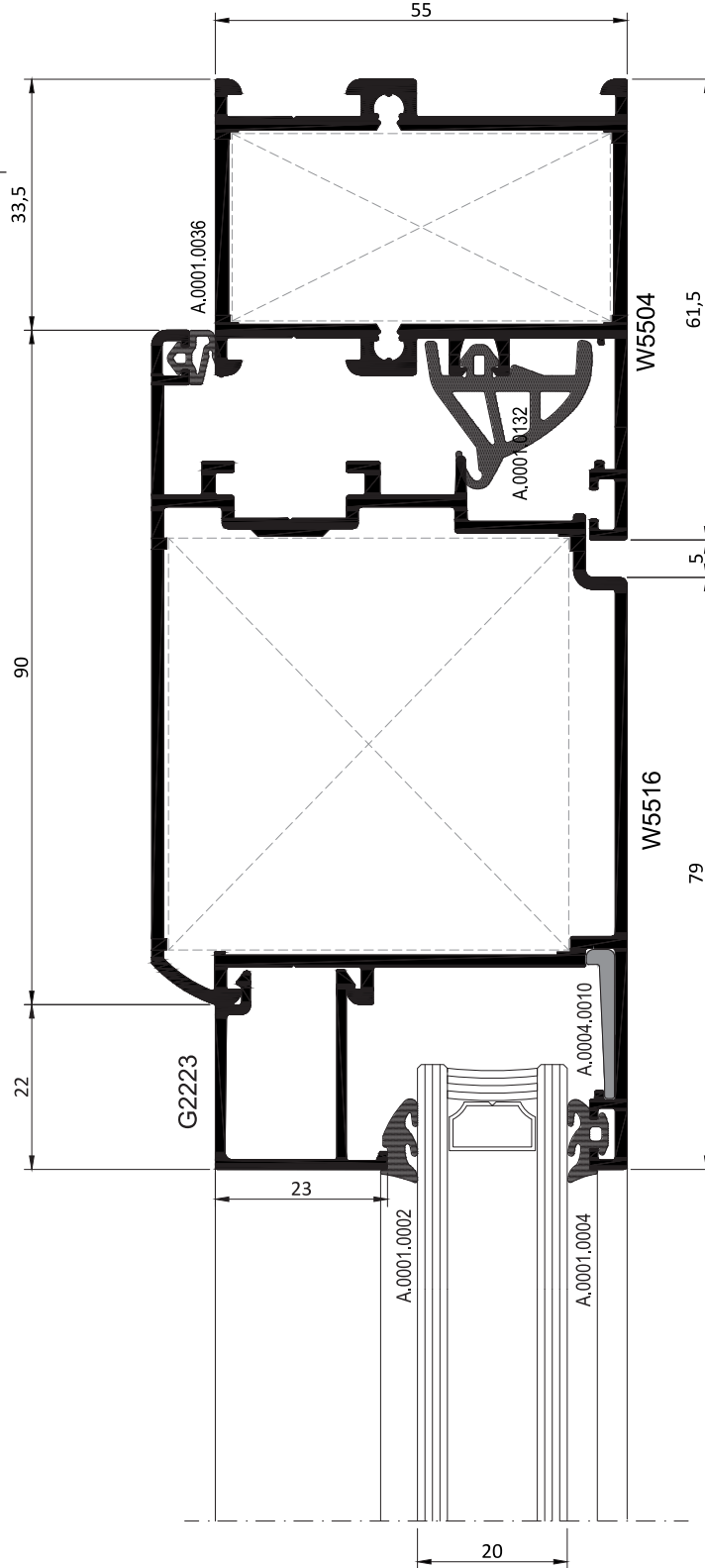
İÇE AÇILIM BİNLİ KAPI DETAYI INWARD OPENING DOOR DETAIL
