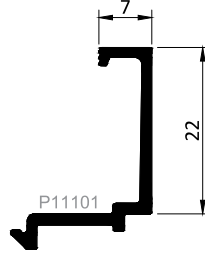
Kod / Code : G2207 Profil No / Profile No : P11101 Ağırlık / Weight : 0.198 kg/m
