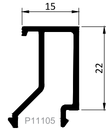
Kod / Code : G2215 Profil No / Profile No : P11105 Ağırlık / Weight : 0.264 kg/m
