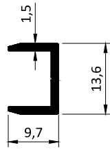
Kod / Code : WT6454 Profil No / Profile No : P13051 Ağırlık / Weight : 0.117 kg/m
