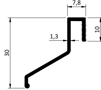
Kod / Code : - Profil No / Profile No : 10150 Ağırlık / Weight : 0.198 kg/m
