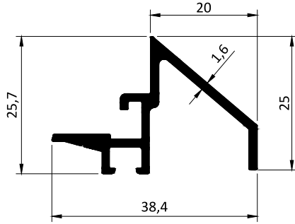
Kod / Code : WT6452 Profil No / Profile No : P13049 Ağırlık / Weight : 0.385 kg/m
