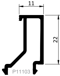
Kod / Code : G2211 Profil No / Profile No : P11103 Ağırlık / Weight : 0.257 kg/m
