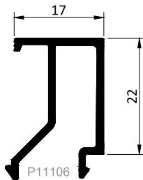
Kod / Code : G2217 Profil No / Profile No : P11106 Ağırlık / Weight : 0.270 kg/m
