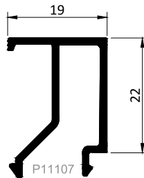
Kod / Code : G2219 Profil No / Profile No : P11107 Ağırlık / Weight : 0.277 kg/m
