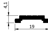
Kod / Code : - Profil No / Profile No : 10151 Ağırlık / Weight : 0.122 kg/m
