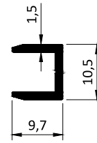
Kod / Code : WT6455 Profil No / Profile No : P13052 Ağırlık / Weight : 0.104 kg/m
