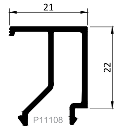
Kod / Code : G2221 Profil No / Profile No : P11108 Ağırlık / Weight : 0.283 kg/m
