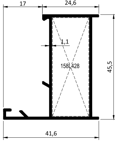
Kod / Code : W4501 Profil No / Profile No : P11300 Ağırlık / Weight : 0.502 kg/m
