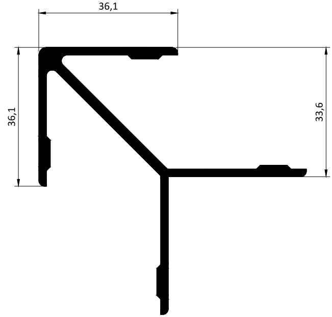
Kod / Code : L0336 Profil No / Profile No : P11011 Ağırlık / Weight : 1.157 kg/m
