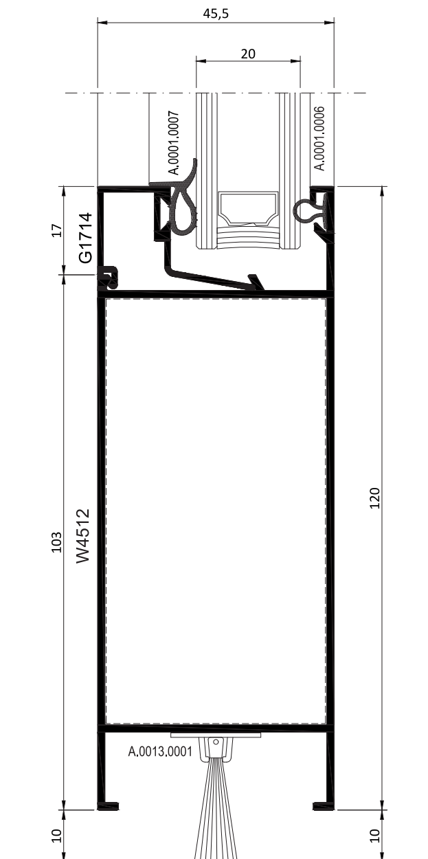
ÇİFT KANAT KAPI DOUBLE VENT DOOR
