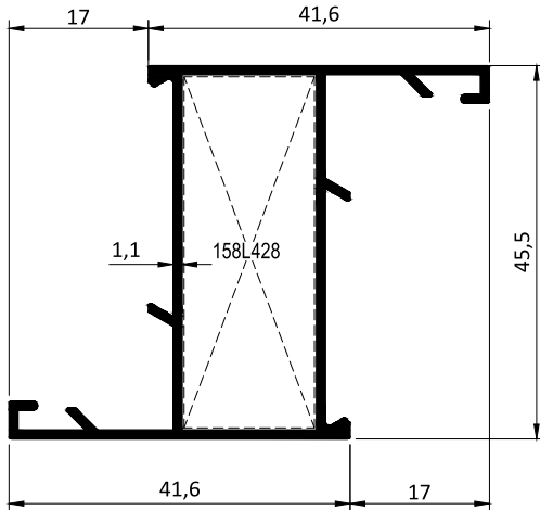
Kod / Code : W4503 Profil No / Profile No : P11302 Ağırlık / Weight : 0.599 kg/m
