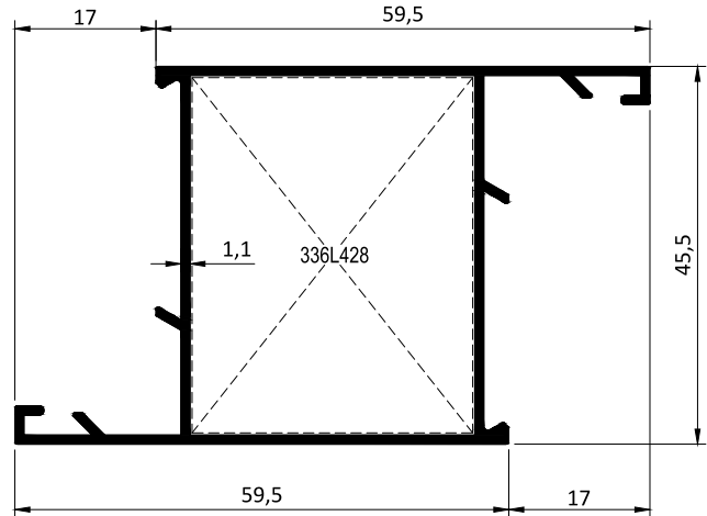
Kod / Code : W4504 Profil No / Profile No : P11303 Ağırlık / Weight : 0.706 kg/m
