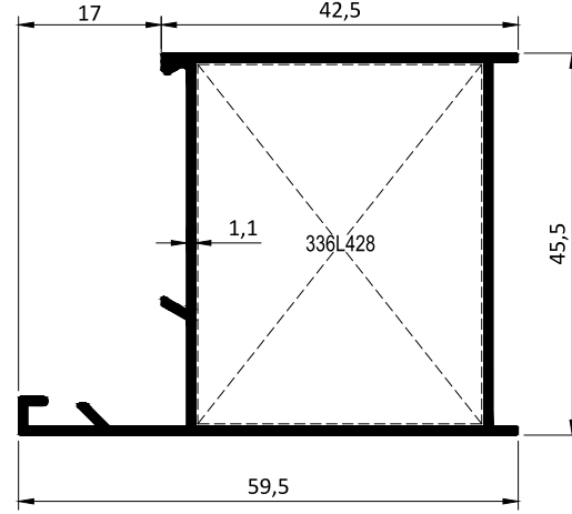
Kod / Code : W4502 Profil No / Profile No : P11301 Ağırlık / Weight : 0.608 kg/m
