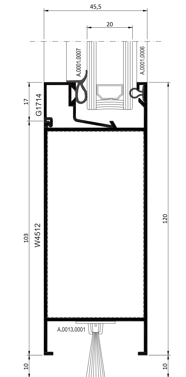
ÇARPMA KAPI SWINGING DOOR
