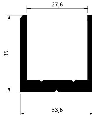
Kod / Code : T0336 Profil No / Profile No : P11317 Ağırlık / Weight : 0.967 kg/m
