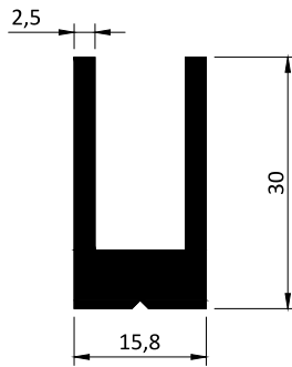
Kod / Code : T0158 Profil No / Profile No : P11316 Ağırlık / Weight : 0.608 kg/m
