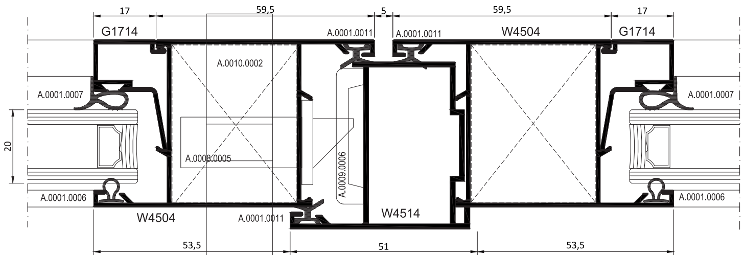
ÇİFT KANAT KAPI DOUBLE VENT DOOR
