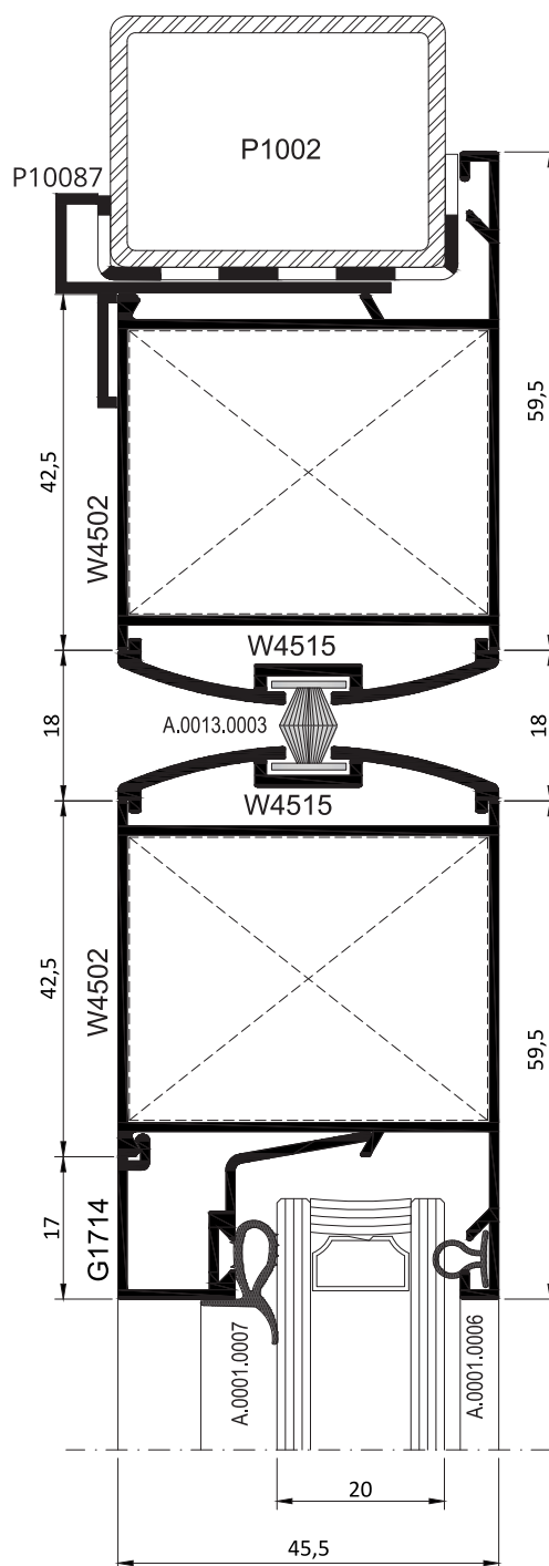
ÇARPMA KAPI SWINGING DOOR
